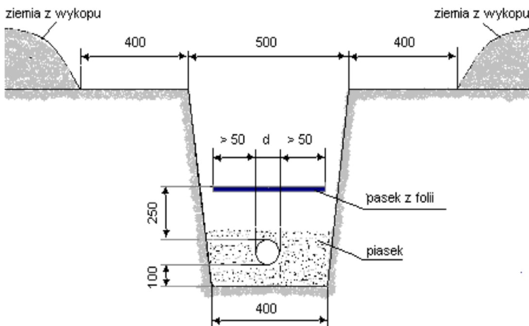
Ryc. 5. Przykładowy rów kablowy - kabel przykryty folią z tworzywa sztucznego (wymiarzy podane w mm).
