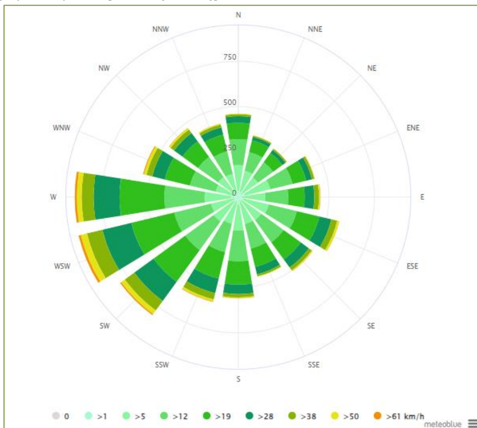
Rysunek 41. Róża wiatrów na terenie Miasta Mława. Źródło: meteoblue.com
