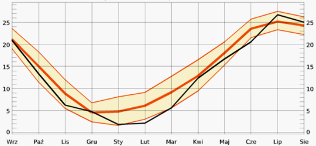
Rysunek 46. Porównanie klimatyczne: miesięczna średnia temperatura powietrza. Ostatnie 12 miesięcy (sierpień 2022 – wrzesień 2023) – czarna linia oraz 30-letni klimat dla Miasta Mława.
